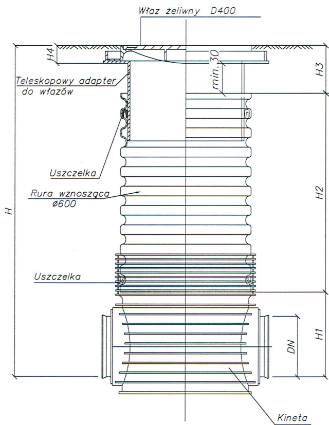
Studzienka kanalizacyjna ø600
